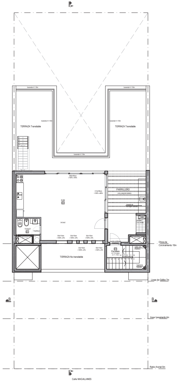
PLANTA NIVEL 11 Esc 1:100
