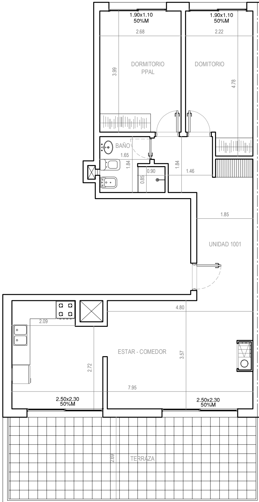
UNIDAD 1001 100.PISO AL FRENTE
